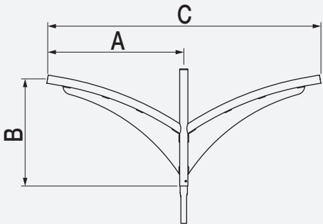
crosse Delphi double feu
