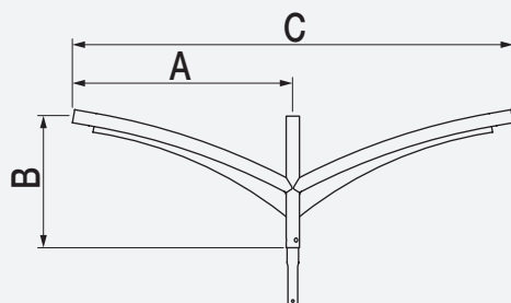
crosse Cytise double feu
