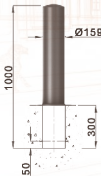
Borne encastrée
